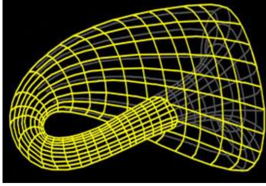
Şekil 001 : Klein şişesi
